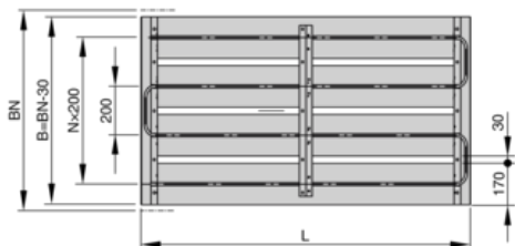
Abb. 2: WK-D-WF mit mittlerem Z-Winkel ( L > 2500 mm)
