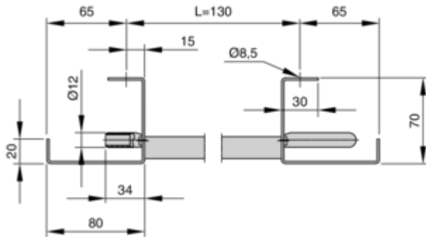
Abb. 9: WK-D-WF Abdeck-/Aufhängewinkel - Länge <math>< 2500\text{ mm}</math>
