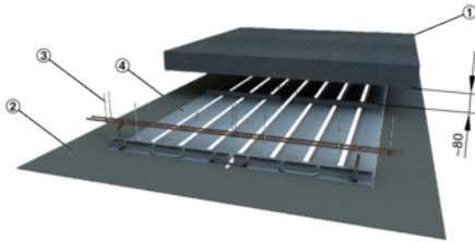
Abb. 6: Kühldeckenelement in geschlossenen Decken integriert
