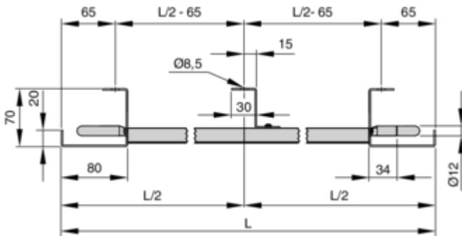
Abb. 10: WK-D-WF Abdeck-/Aufhängewinkel - Länge <math>\ge 2500\text{ mm}</math>
