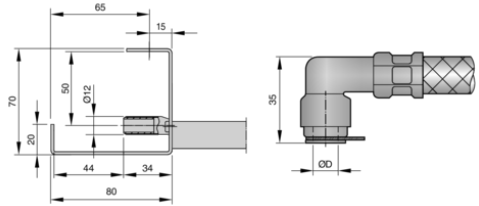
Abb. 8: WK-D-WF Anschlussituation
