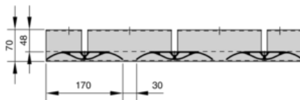
Abb. 3: WK-D-WF Schnitt über Breite
